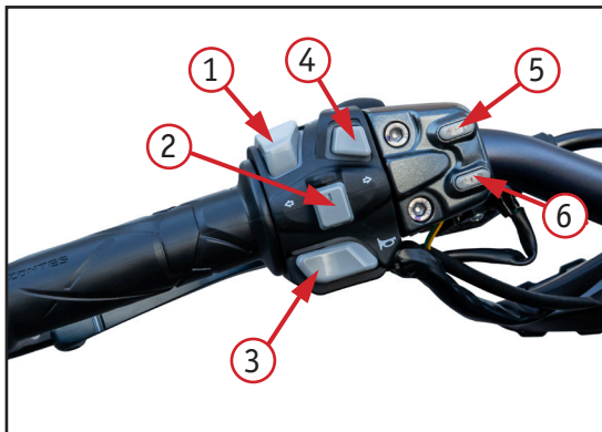
Фото 2.4 Левый комбинированный переключатель: 1 – переключатель режима света фары (дальний свет/ ближний свет); 2 – клавиша указателей поворота; 3 – кнопка звукового сигнала; 4 – кнопка аварийной сигнализации; 5 – кнопка «MOD»; 6 – кнопка «SET»; 7 – кнопка включения дальнего света при обгоне
