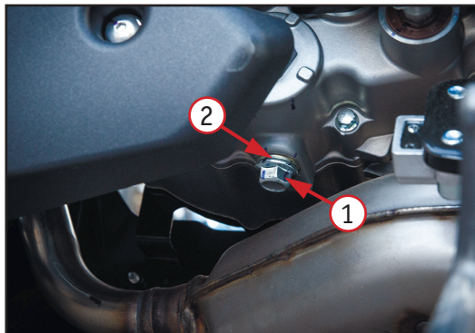
Фото 4.5. Слив моторного масла: сливной болт – 1; шайба – 2
