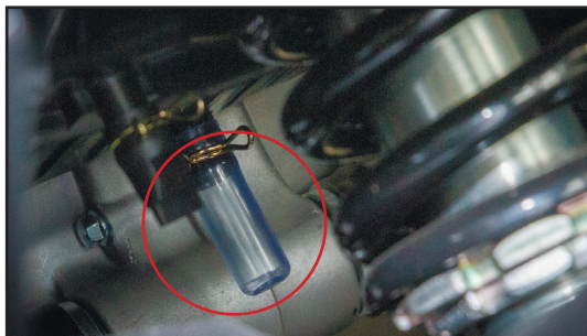
Фото 4.2. Расположение трубки слива масла из отсека воздушного фильтра
