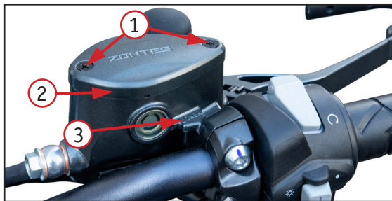
4.8.1. Бачок тормозной жидкости передних тормозов: 1 – винты крепления крышки бачка; 2 – крышка бачка; 3 – уровень «минимум»
