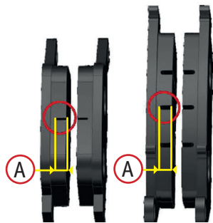
Фото 4.11 Износ тормозных колодок «А»
