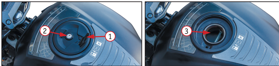
Фото 3.7. Топливный бак: 1 – защитная створка (язычок); 2 – замочная скважина; 3 – заливная горловина
