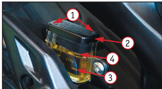
4.8.2. Бачок тормозной жидкости задних тормозов: 1 – винты крепления крышки бачка; 2 – крышка бачка; 3 – уровень «минимум»; 4 – уровень «максимум»
