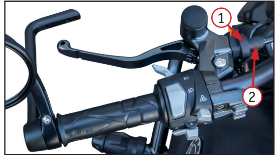
Фото 3.4. Регулировка рычага сцепления на руле 1 – стопорная гайка; 2 – регулировочная гайка
