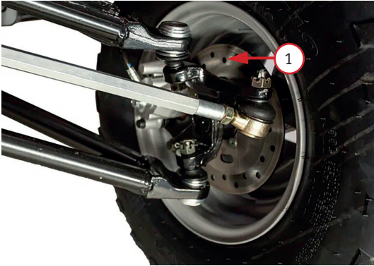
Фото 3.3. Проверка переднего тормозного диска 1
