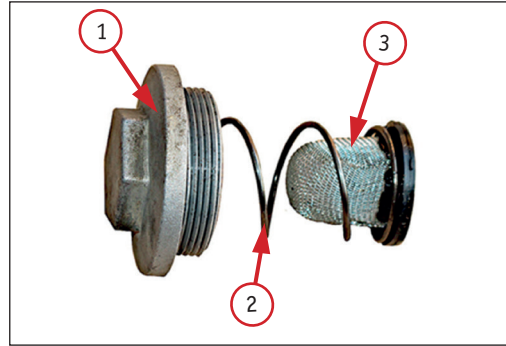
Фото 5.2. Крышка 1 с пружиной 2 и масляным фильтром-сеткой 3
