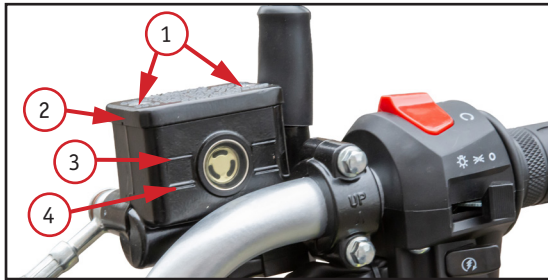
5.11. Бачок тормозной жидкости передних тормозов: 1 – винты крепления крышки бачка; 2 – крышка бачка; 3 – уровень «максимум»; 4 – уровень «минимум»
