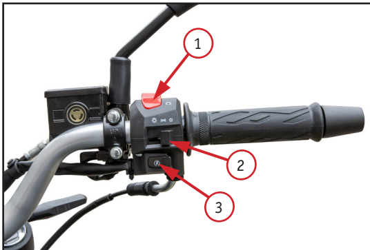
Фото 2.5.1. Правый комбинированный переключатель для моделей BATLLO, CARRERA: 1 – переключатель включения/отключения зажигания; 2 – переключатель освещения; 3 – кнопка электростартера
