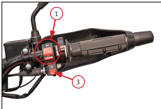
Фото 2.5.2. Правый комбинированный переключатель для модели CROSSER: 1 – переключатель включения/отключения зажигания; 3 – кнопка электростартера
