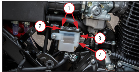
5.12. Бачок тормозной жидкости задних тормозов: 1 – винты крепления крышки бачка; 2 – крышка бачка; 3 – уровень «максимум»; 4 – уровень «минимум»
