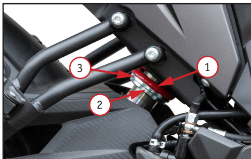
Фото 5.15. Регулировка преднатяга амортизатора: 1 – пружина; 2 – стопорная гайка, 3 – регулировочная гайка
