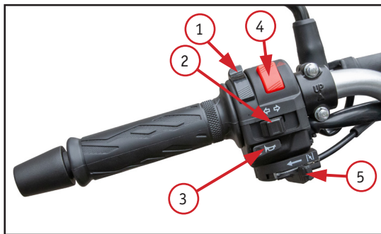
Фото 2.4.1 Левый комбинированный переключатель для моделей BATLLO, CARRERA: 1 – переключатель режима света фары (дальний свет/ ближний свет); 2 – клавиша указателей поворота; 3 – кнопка звукового сигнала; 4 – кнопка аварийной сигнализации; 5 –рычаг воздушной заслонки (обоганитель топливной смеси) (только для модели BATLLO); 6 – кнопка включения дальнего света при обгоне
