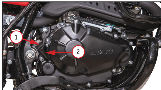
Фото 5.2.2. Контроль уровня масла для моделей CARRERA и CROSSER: 1 – щуп контроля уровня масла; 2 – заливная горловина
