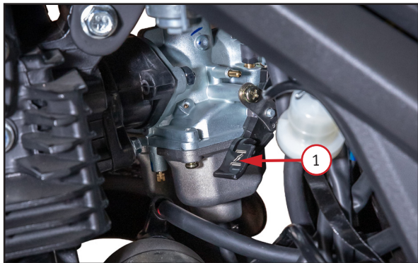
Фото 3.2. Рычаг воздушной заслонки (обогащения топливной смеси) – 1 для моделей CARRERA и CROSSER
