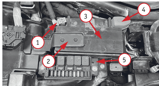
Фото 4. Аккумуляторный отсек: 1 – клемма «минус»; 2 – крепление аккумуляторной батареи (АКБ); 3 – аккумуляторная батарея; 4 – колпачок клеммы «плюс»; 5 – блок предохранителей
