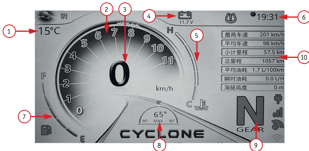
Фото 2.9. Приборная TFT-панель: 1 – температура окружающей среды; 2 – шкала тахометра; 3 – показатель скорости; 4 – заряд АКБ; 5 – шкала температуры охлаждающей жидкости; 6 – текущее время; 7 – уровень топлива в баке; 8 – температура двигателя; 9 – текущая передача; 10 – переменные показатели (средняя скорость, общий километраж пробега, расход топлива и др.)
