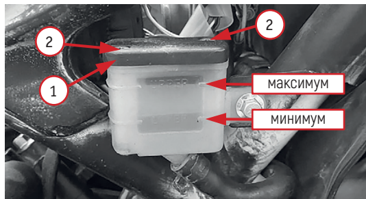
Фото 5.8.1. Бачок тормозной жидкости задних тормозов: 1 – крышка бачка; 2 – винты крепления крышки бачка
