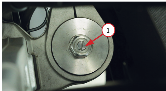
Фото 2.13. Регулировка демфирования переднего амортизатора: регулировочный винт - 1
