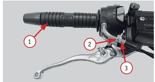
Фото 3. Регулировка троса газа: 1 – ручка газа (акселератора); 2 – стопорная гайка; 3 – регулировочная гайка
