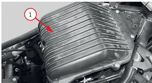
Фото 5.1. Снятие воздушного фильтра: 1 – крышка отсека воздушного фильтра; 2 – фильтрующий элемент
