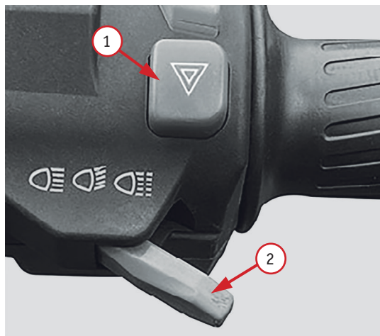
Фото 2.3. Левый комбинированный переключатель: 1 – кнопка включения аварийных сигналов; 2 – переключатель света фары (дальний/ближний/дальний при обгоне); 3 – клавиша «MODE»; 4 - клавиша «SET»; 5 - клавиша «ENT»; 6 – переключатель указателя поворотов; 7 – кнопка звукового сигнала; 8 – кнопка подъема ветрового стекла; 9 – кнопка включения прожектора; 10 – кнопка опускания ветрового стекла
