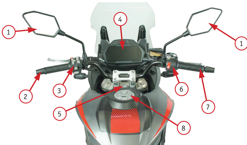
Фото 2.1. Вид руля и органов управления мотоцикла: 1- зеркало заднего вида; 2 - левая рулевая рукоятка; 3 - левый комбинированный переключатель; 4 - приборная панель; 5 - кнопка включения/отключения зажигания; 6 - правый комбинированный переключатель; 7 - рукоятка газа (акселератор); 8 - крышка топливного бака
