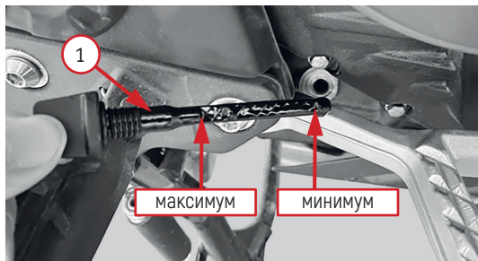
Фото 5.4. Пробка с щупом контроля уровня масла 1
