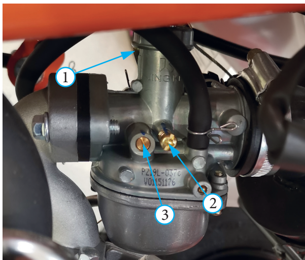
Фото 5.5 Регулировка карбюратора:
