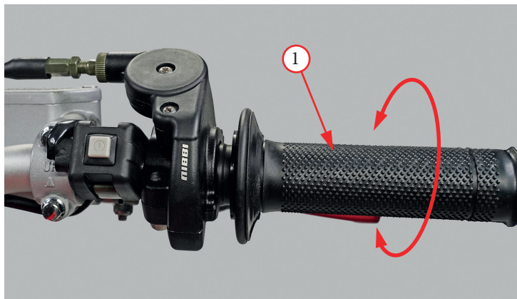
Фото 3.5.1. Ручка акселератора – 1
