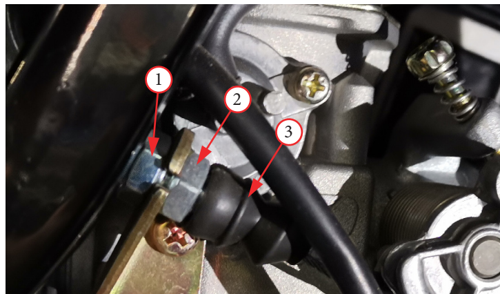
Фото 26. Регулировка хода троса акселератора в моторном отделении модели WD 150.
