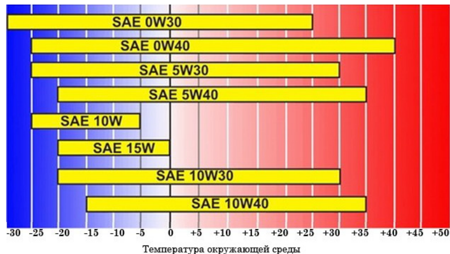
Рисунок 16. Схема для выбора моторного масла.
