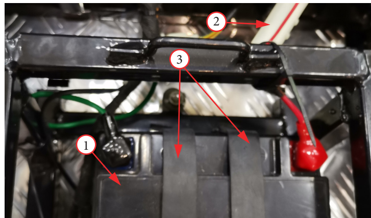
Фото 12. Снятие аккумуляторной батареи.
