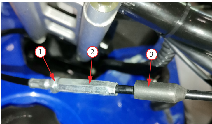
Фото 25. Регулировка хода троса акселератора на моделях WD 150 и WD 160
