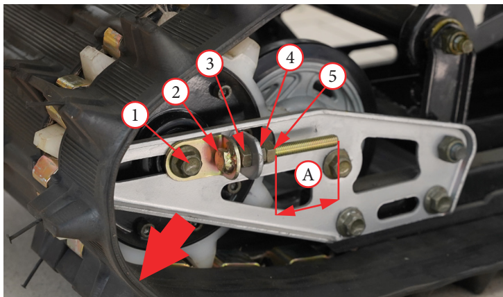
Фото 24.1 Регулировка гусеницы на модели WD150.
