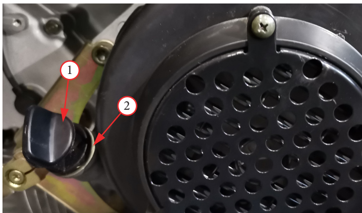
Фото 17. Проверка уровня масла в двигателе.
