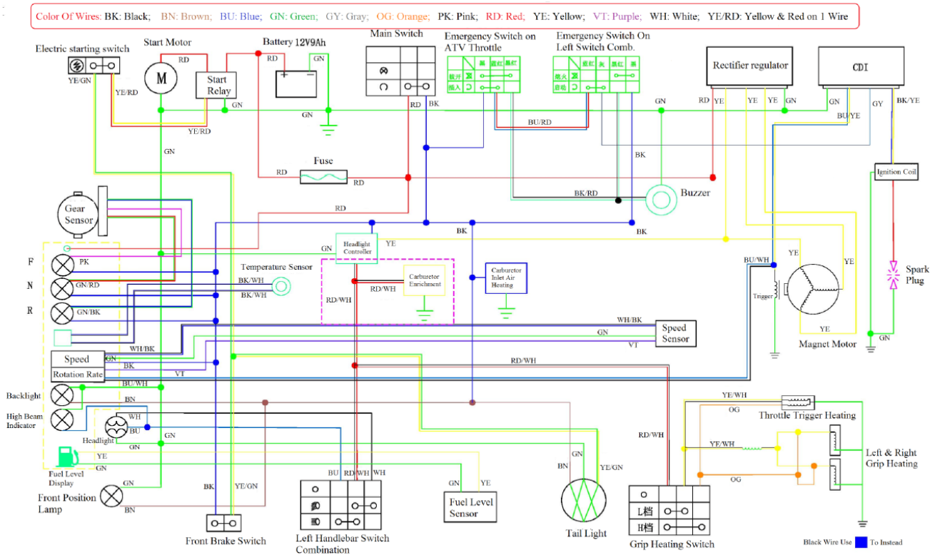
Схема 1. Электрическая схема снегохода WD150.
