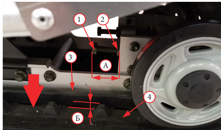
Фото 24.2 Регулировка гусеницы на модели WD160.
