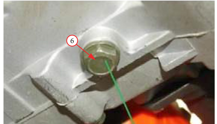
Фото 19. Замена масла в редукторе.
