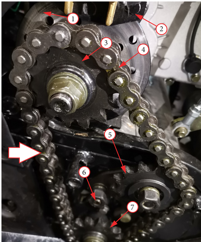
Фото 22. Проверка и регулировка цепи.
