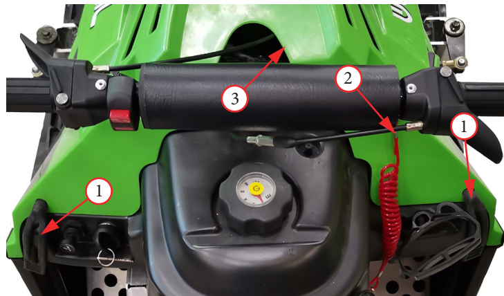
Фото 11. Снятие сиденья на модели WD160: 1 – резиновые ремни крепления; 2 – кабель с пластмассовым штифтом; 3 – крышка моторного отсека.
