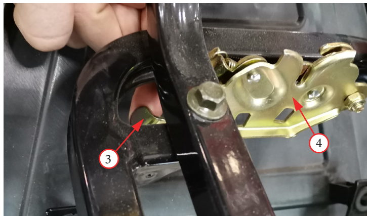
Фото 10. Снятие сиденья на модели WD150: 1 – болт; 2 – задняя крышка сиденья; 3 – рычаг фиксатора замка; 4 – замок.
