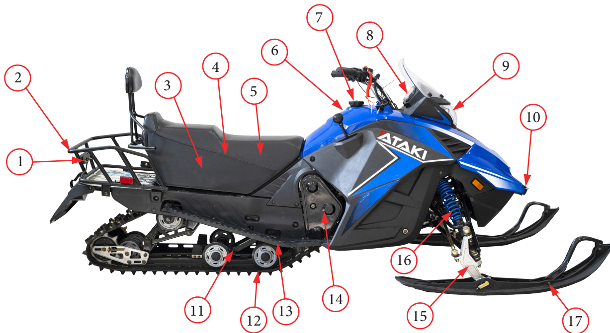
Фото 2.1 Узлы и части снегохода модели WD150: 1 - задний фонарь; 2 - задний багажник; 3 – сиденье (под сиденьем: 4 – предохранитель и электрические компоненты; 5 – аккумулятор); 6 – рукоятка ручного запуска (с левой стороны); 7 – карбюратор (с левой стороны за обвесом); 8 – приборная панель; 9 – фара; 10 - передний бампер; 11 - узел задней подвески с роликами; 12 - резиновая гусеница; 13 – подножка водителя; 14 – цепная передача (за крышкой); 15 – поворотный кулак; 16 – амортизатор; 17 - лыжа.
