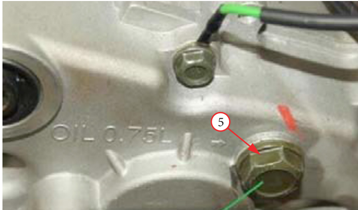
Фото 19. Замена масла в редукторе.
