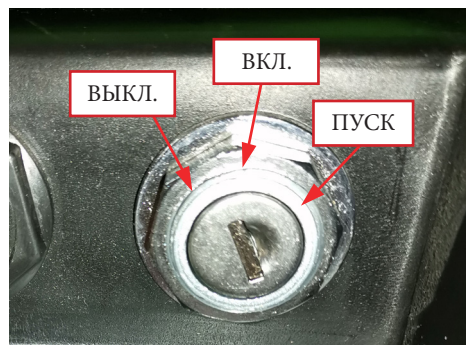
Фото 3.2. Замок зажигания модели WD160.
