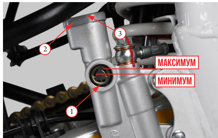
Фото 5.17. Контроль и долив тормозной жидкости
