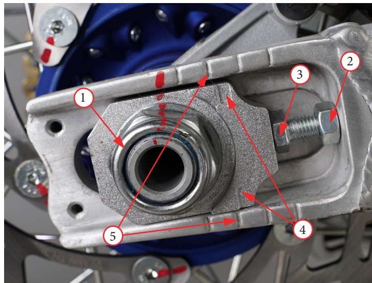
Фото 5.25. Регулировка натяжения цепи
