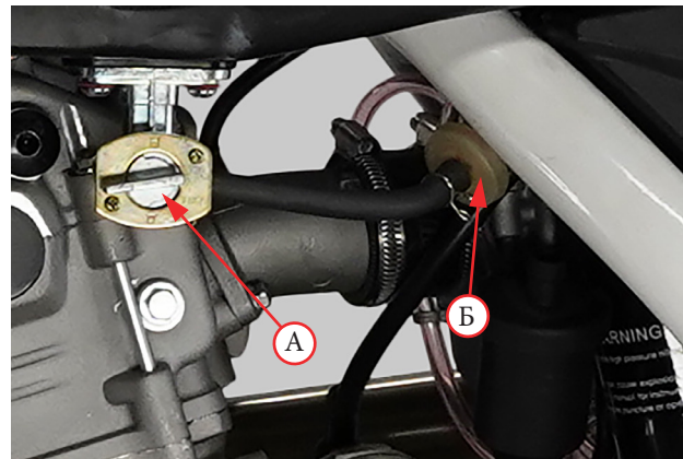
Фото 3.2. Места установки: А-топливный кран; Б- топливный фильтр
