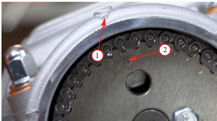
Фото 5.33. Совмещение риски в окне со звездой распределительного вала: 1 – метка на корпусе; 2 – метка «О» на звезде.
