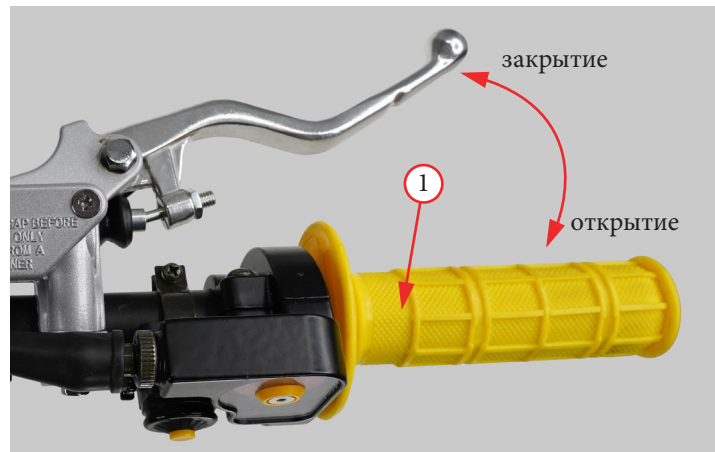
Фото 3.5. Ручка акселератора - 1
