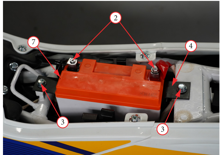
Фото 5.7. Снятие аккумуляторной батареи
