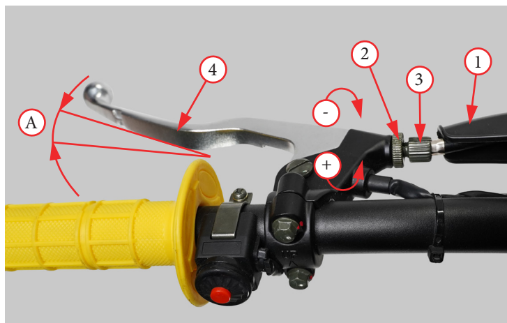
Фото 5.10. Регулировка свободного хода рычага сцепления (варианты исполнения)
