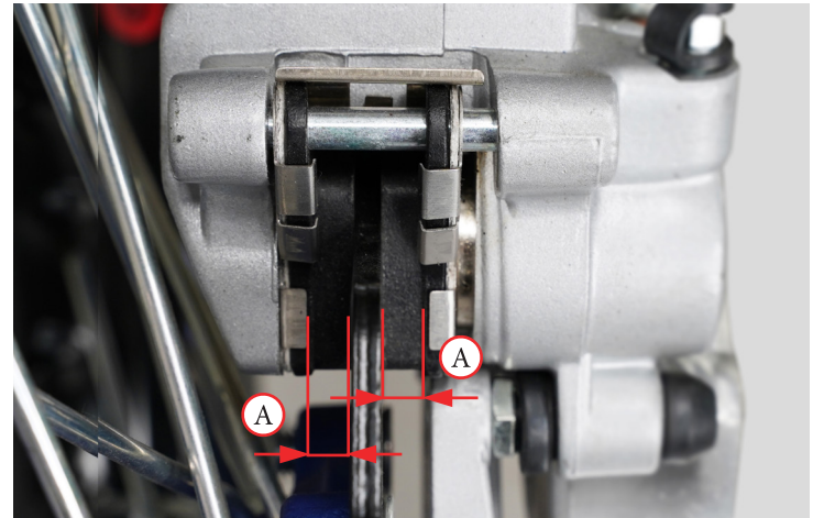
Фото 5.18 Контроль тормозных колодок
