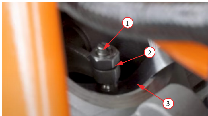
Фото 5.34. Регулировки теплового зазора: 1 – регулировочный винт; 2 – контргайка; 3 – щуп.
