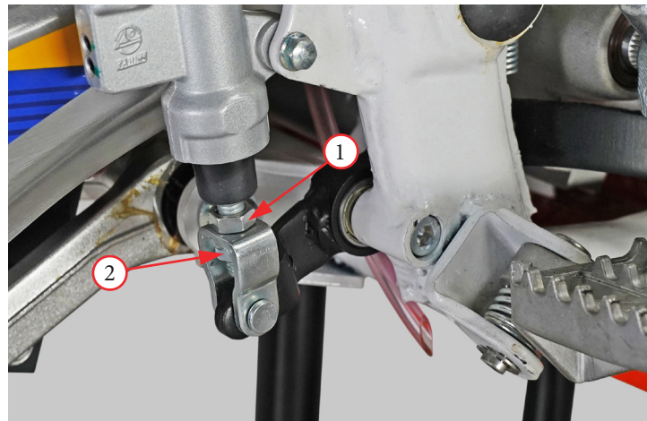
Фото 5.16. Регулировка высоты педали заднего тормоза
