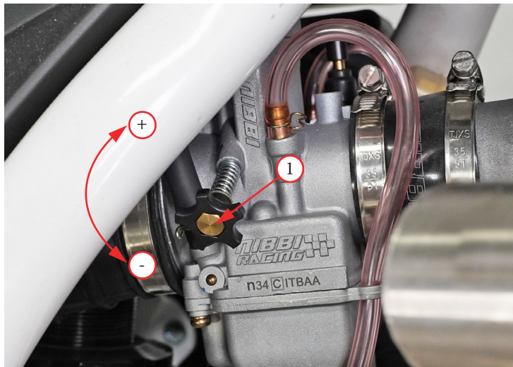
Фото 5.9. Регулировка холостых оборотов
