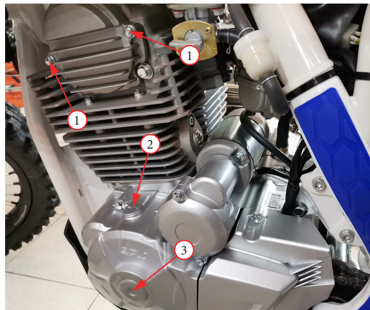
Фото 5.30. Крышки окон левой стороны двигателя: 1 – болты крепления крышки распределительного вала; 2 – крышка смотрового окна; 3 – крышка доступа к коленчатому валу.
