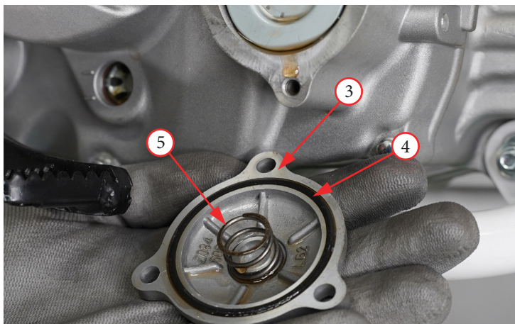
Фото 5.3. Замена масла в двигателе ZS174MN
