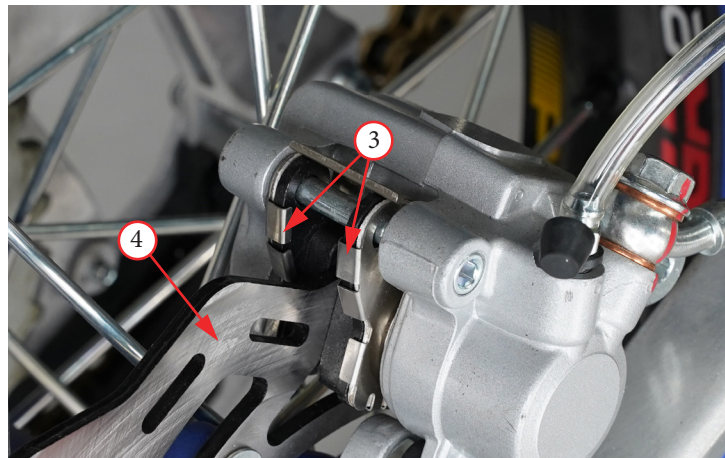
Фото 5.21. Замена задних тормозных колодок
