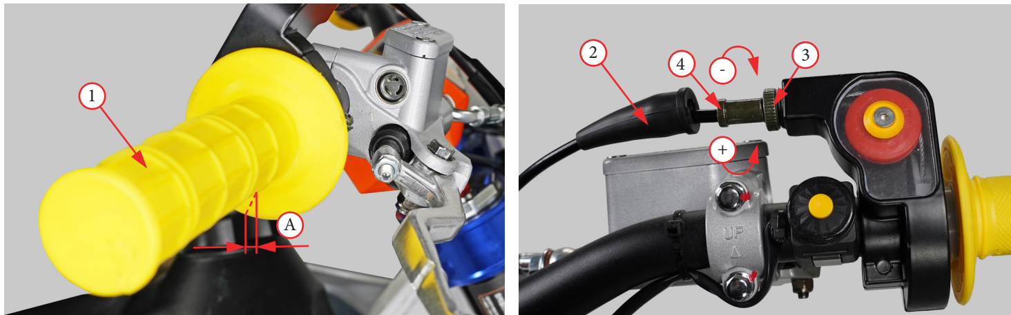
Фото 5.8. Регулировка свободного хода рукоятки акселератора
