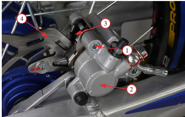
Фото 5.21. Замена задних тормозных колодок
