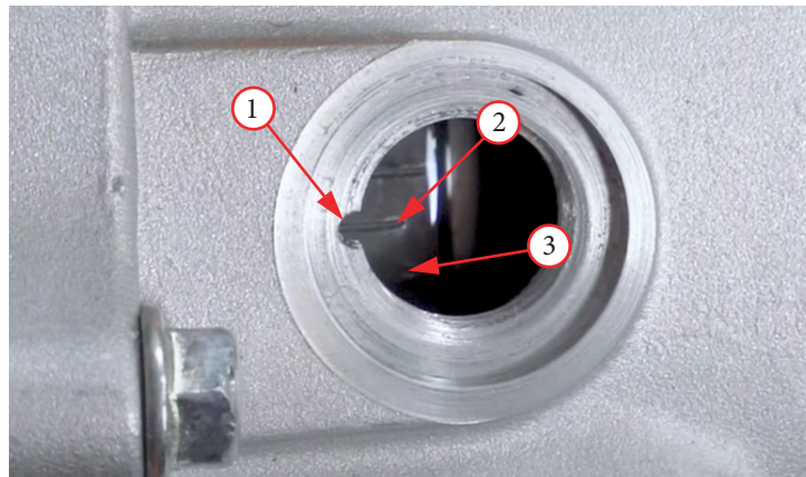
Фото 5.32. Совмещение риски на боковом окне с меткой на валу: 1 – выточка на окне; 2 – метка на маховике; 3 – метка «Т».
