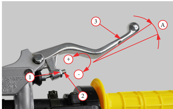
Фото 5.15 Регулировка передних тормозов
