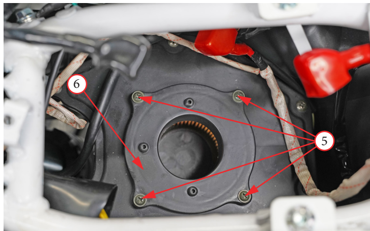
Фото 5.7.1 Снятие воздушного фильтра
