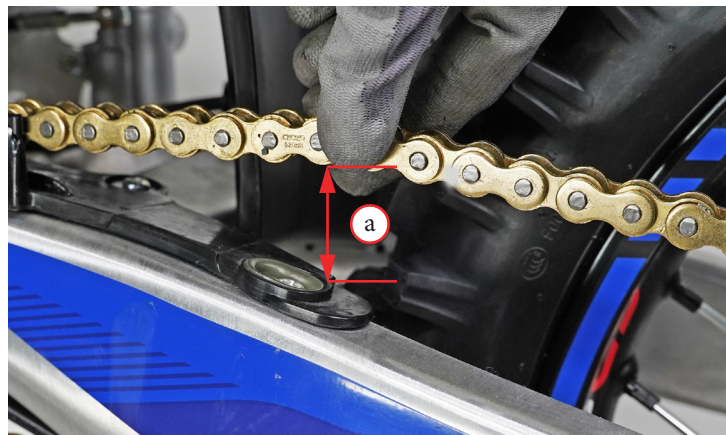
Фото 5.22. Замер провисания цепи
