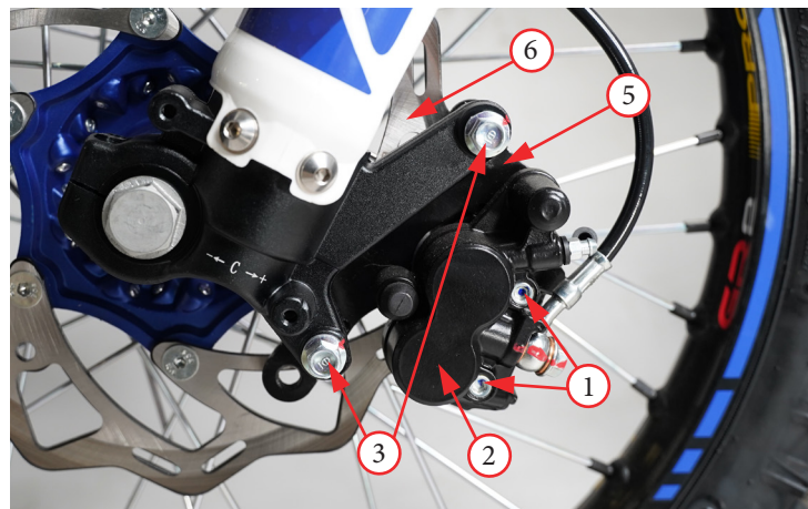
Фото 5.20. Замена передних тормозных колодок
