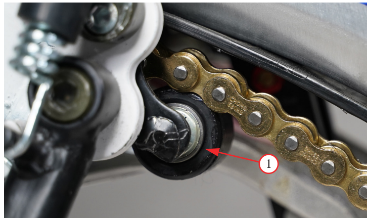
Фото 5.24. Ролик натяжения цепи
