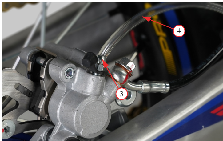
Фото 5.19. Подсоединение трубки к штуцеру
