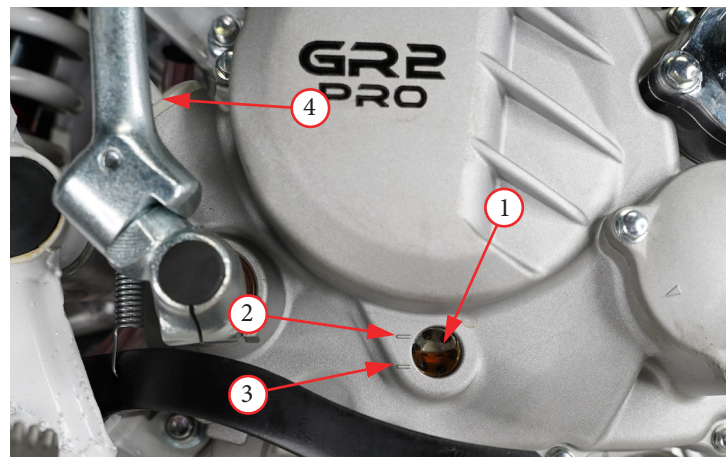
Фото 5.2. Варианты исполнения смотрового окна и крышки горловины двигателей ZS172FMM, ZS174MM: 1 - смотровое окно с указателями уровня (максимум - «2» и минимум - «3»); 4 - крышка маслозаливной горловины.
