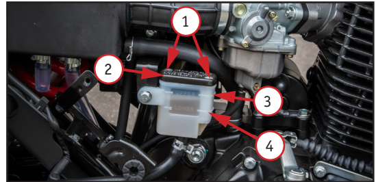
5.12. Бачок тормозной жидкости задних тормозов для моделей BATLLO, CARRERA, CROSSER: 1 – винты крепления крышки бачка; 2 – крышка бачка; 3 – уровень «максимум»; 4 – уровень «минимум»
