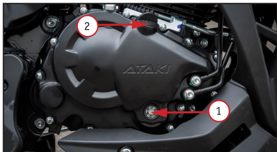
Фото 5.2.1. Контроль уровня масла для модели BATLLO: 1 – смотровое окно; 2 – крышка заливной горловины
