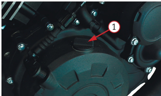
Фото 5.4. Пробка горловины для залива масла – 1
