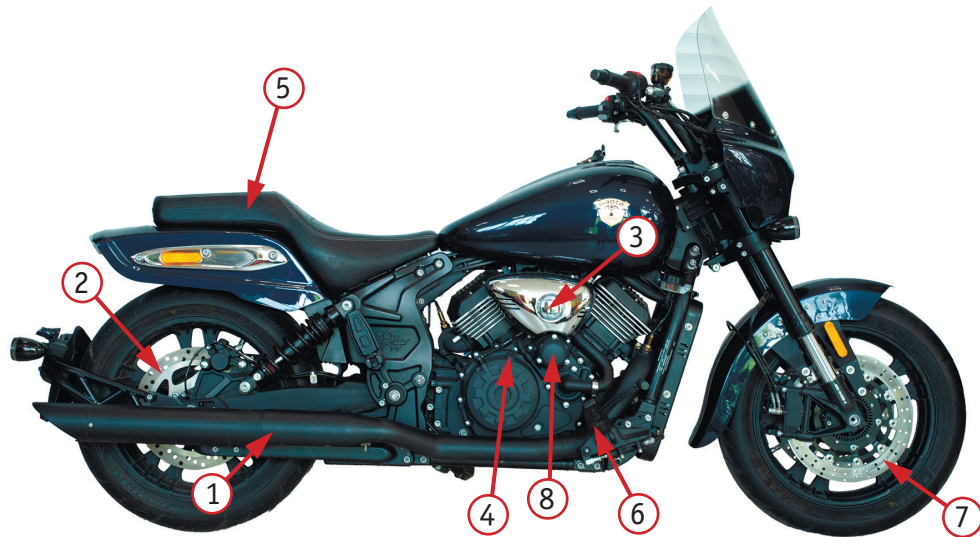
Фото 2.2. Вид справа: 1 – глушитель; 2 – задние дисковые тормоза; 3 – замок зажигания; 4 – заливная горловина для масла; 5 – сиденье; 6 – подножка водителя; 7 – передние дисковые тормоза; 8 – крышка масляного фильтра
