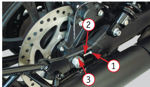
Фото 5.8 Регулировка ремня: 1 - регулировочная гайка; 2 - стопорная гайка; 3 - гайка задней оси
