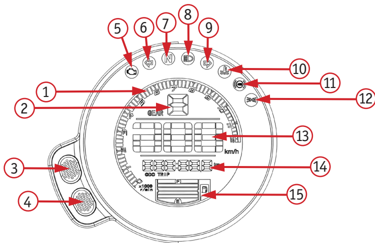
Фото 2.12. Вид приборной панели модели SL800: 1 – тахометр; 2 – индикатор передачи; 3 – кнопка «Вверх»; 4 – кнопка «Вниз»; 5 – индикатор неисправности EFI; 6 – индикатор левого поворотника; 7 – индикатор нейтральной передачи; 8 – индикатор дальнего света; 9 – индикатор правого поворотника; 10 – индикатор перегрева двигателя; 11 – индикатор ABS; 12 – индикатор габаритных огней; 13 – скорость; 14 – общий/текущий пробег; 15 – количество топлива
