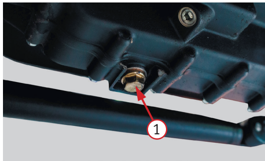
Фото 5.5. Болт слива масла – 1
