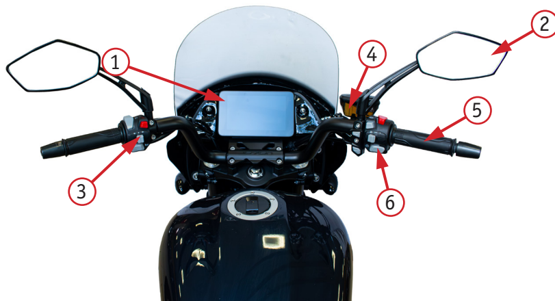
Фото 2.1. Вид руля и органов управления мотоцикла: 1 – приборная панель; 2 – зеркало заднего вида; 3 – левый комбинированный переключатель; 4 – бачок для тормозной жидкости; 5 – рукоятка газа (акселератор); 6 – правый комбинированный переключатель
