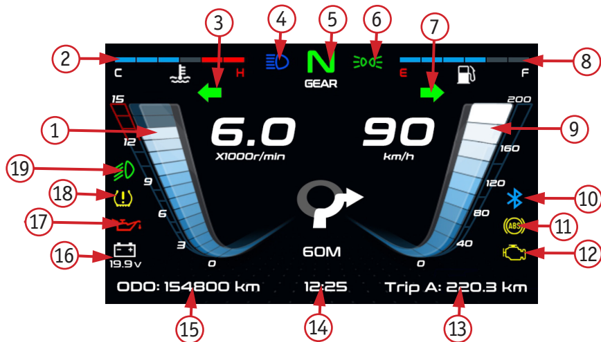
Фото 2.10. Вид приборной панели моделей ML800 и RL800: 1 – тахометр; 2 – температура двигателя; 3 – индикатор левого поворотника; 4 – индикатор дальнего света; 5 – индикатор передачи; 6 – индикатор габаритных огней; 7 – индикатор правого поворотника; 8 – количество топлива; 9 – скорость; 10 – индикатор подключения Bluetooth; 11 – индикатор ABS; 12 – индикатор неисправности EFI; 13 – текущий пробег; 14 – время; 15 – общий пробег; 16 – напряжение батареи; 17 – индикатор пониженного давления масла; 18 – индикатор пониженного давления в шинах; 19 – индикатор ближнего света
