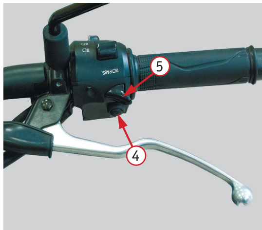
Фото 2.4.2 Левый комбинированный переключатель моделей SL800 и YL800: 1 – кнопка переключения режима света фары (дальний свет/ближний свет); 2 – переключатель указателей поворота; 3 – кнопка звукового сигнала; 4 – кнопка аварийной сигнализации; 5 – кнопка включения дальнего света при обгоне
