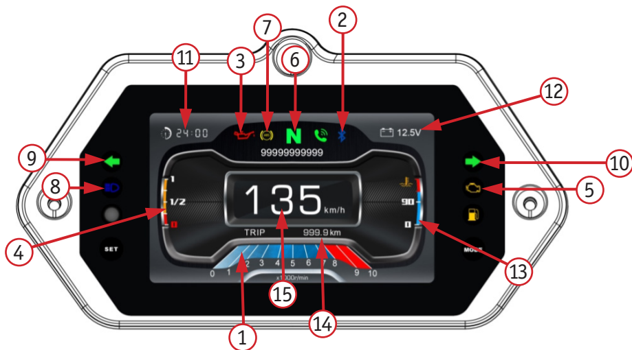
Фото 2.11. Вид приборной панели модели YL800: 1 – тахометр; 2 – индикатор подключения Bluetooth; 3 – индикатор пониженного давления масла; 4 – количество топлива; 5 – индикатор неисправности EFI; 6 – индикатор передачи; 7 – индикатор ABS; 8 – индикатор дальнего света; 9 – индикатор левого поворотника; 10 – индикатор правого поворотника; 11 – время; 12 – напряжение батареи; 13 – температура двигателя; 14 – общий пробег; 15 – скорость
