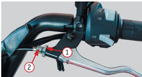
Фото 2.13. Регулировка сцепления: 1 – стопорная гайка; 2 – регулировочный винт
