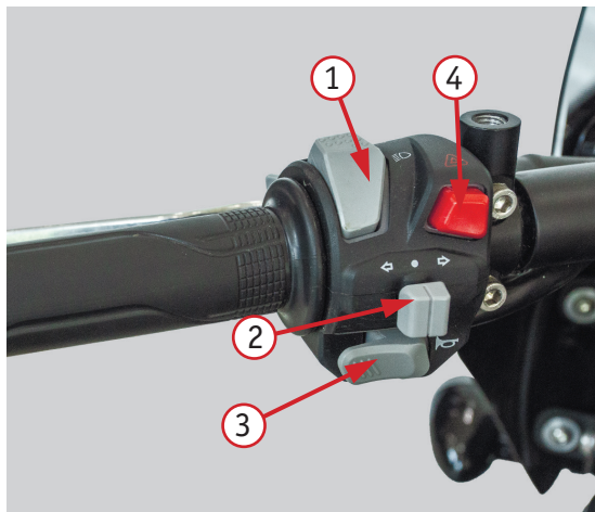
Фото 2.4.1 Левый комбинированный переключатель моделей ML800 и RL800: 1 – кнопка переключения режима света фары (дальний свет/ближний свет); 2 – переключатель указателей поворота; 3 – кнопка звукового сигнала; 4 – кнопка аварийной сигнализации; 5 – кнопка включения дальнего света при обгоне
