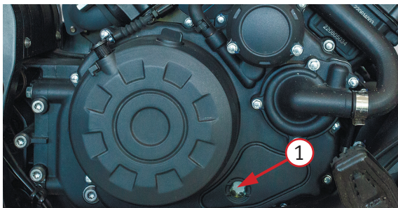
Фото 5.3. Окно для контроля уровня масла – 1
