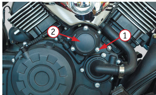
Фото 5.6. Замена масляного фильтра: 1 – винты крышки; 2 – крышка масляного фильтра
