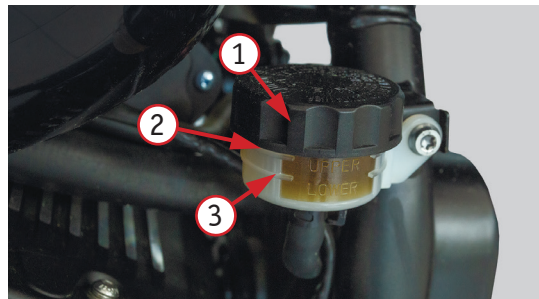
Фото 5.7.2 Уровень тормозной жидкости заднего тормоза: 1 – крышка; 2 – максимум; 3 – минимум
