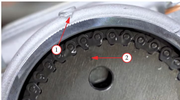
Фото 5.38. Совмещение риски в окне со звездой распределительного вала: 1 – метка на корпусе; 2 – метка «О» на звезде.
