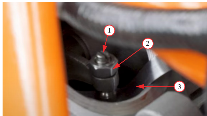
Фото 5.39. Регулировки теплового зазора: 1 – регулировочный винт; 2 – контргайка; 3 – шуп.
