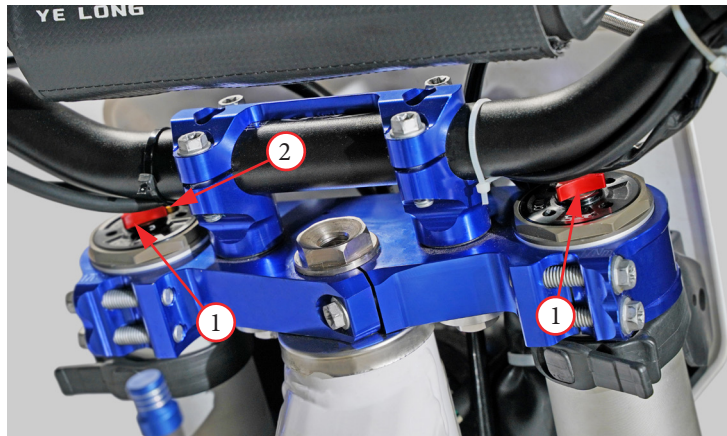
Фото 5.32. Регулировка отбоя передней вилки.
