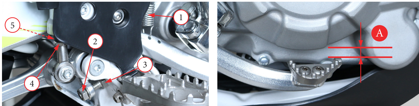
Фото 5.16. Регулировка высоты педали тормоза.
