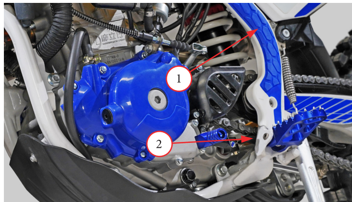
Фото 5.24. Ролик натяжения цепи - 1, слайдер-успокоитель - 2.
