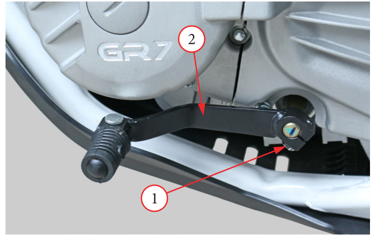
Фото 5.12. Регулировка положения рычага передач.
