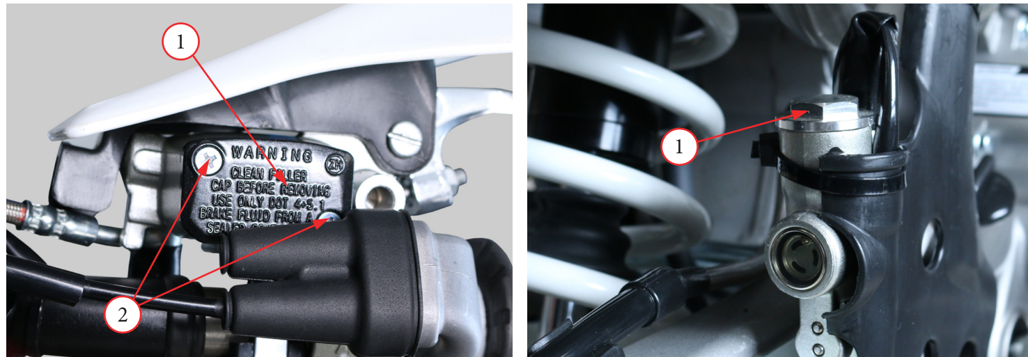
Фото 5.17. Долив тормозной жидкости в контуры.
