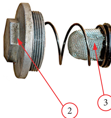
Фото 5.5.3. Замена моторного масла в двигателе с фильтр-сеткой.
