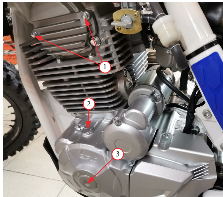
Фото 5.35. Крышки окон левой стороны двигателя: 1 – болты крепления крышки распределительного вала; 2 – крышка смотрового окна; 3 – крышка доступа к коленчатому валу.
