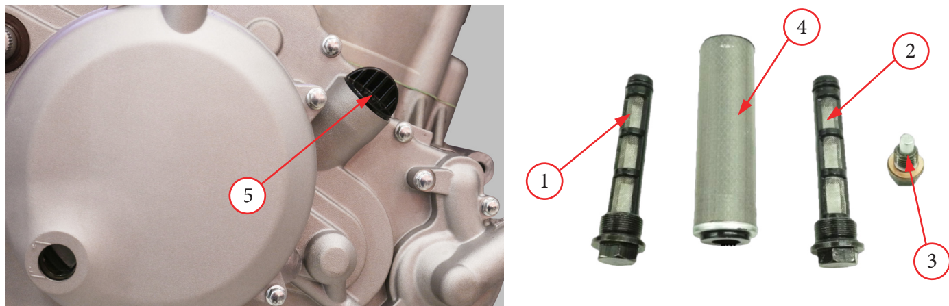
Фото 5.5.2. Части масляного фильтра.
