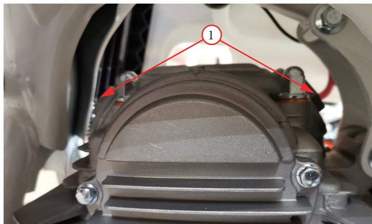
Фото 5.34. Крышки впускного и выпускного клапанов - 1.
