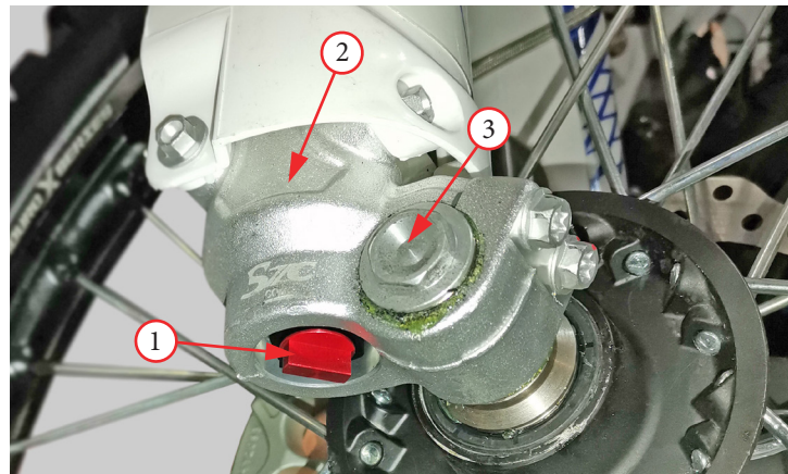
Фото 5.33. Регулировка сжатия передней вилки.
