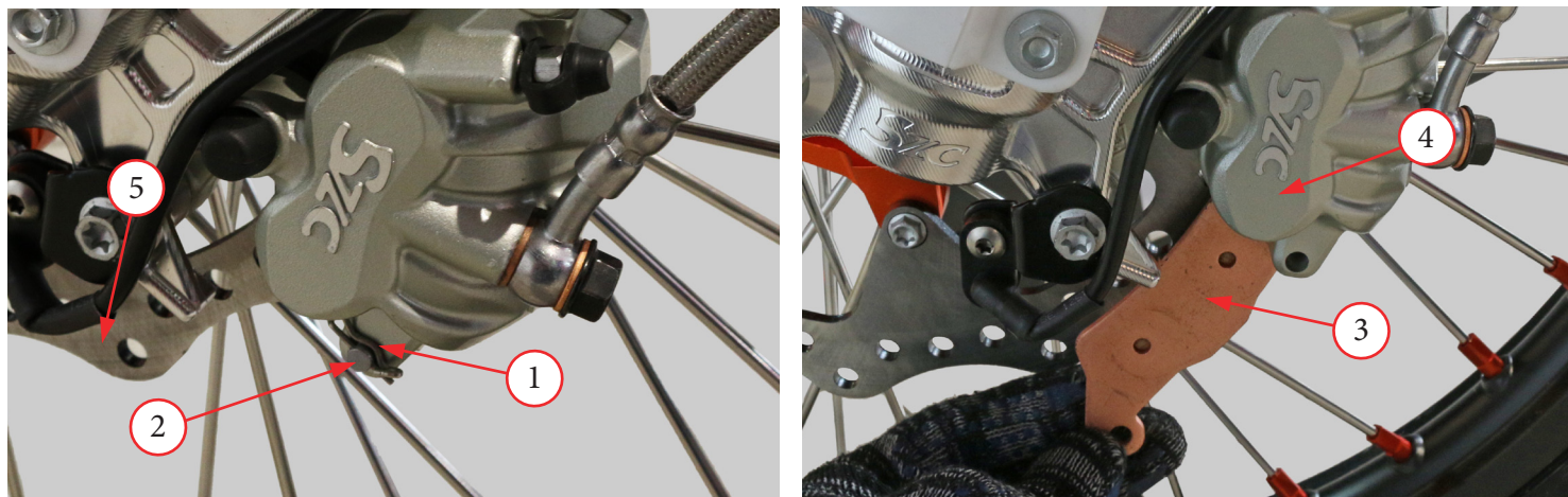
Фото 5.20. Замена передних тормозных колодок.
