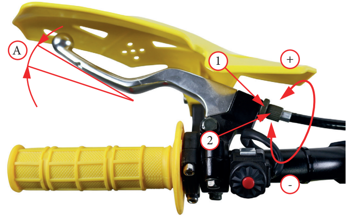
Фото 5.10. Регулировка свободного хода рычага
