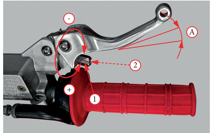
Фото 5.15. Регулировка передних тормозов
