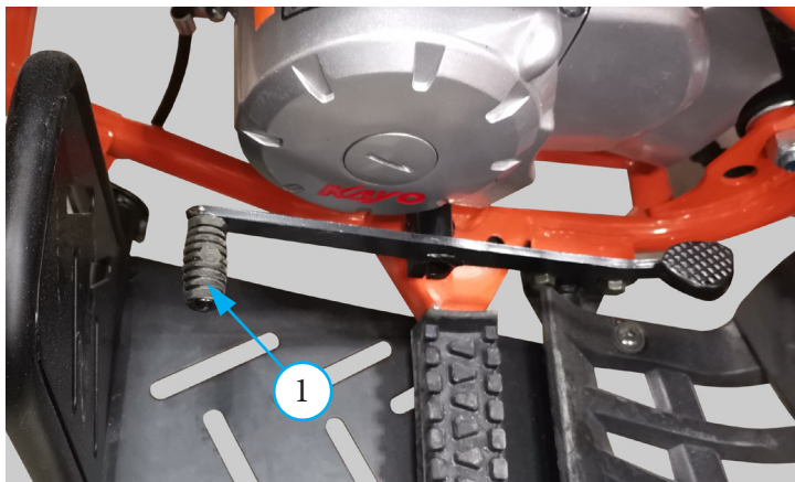
Фото 3.6. Рычаг переключения передач (ножной и ручной).
