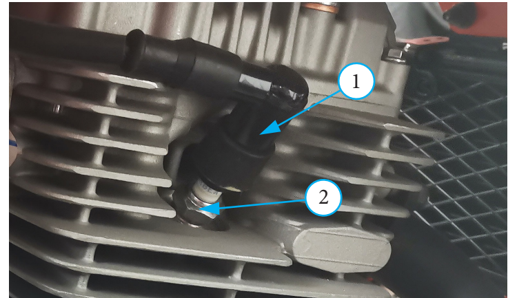
Фото 3.5. Свеча зажигания с колпачком: 1 - колпачок свечи; 2 - свеча зажигания.
