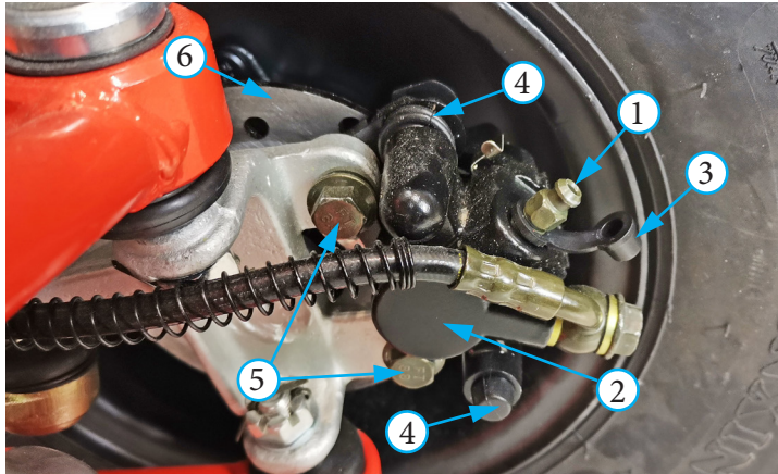
Фото 5.12. Тормозной узел:
