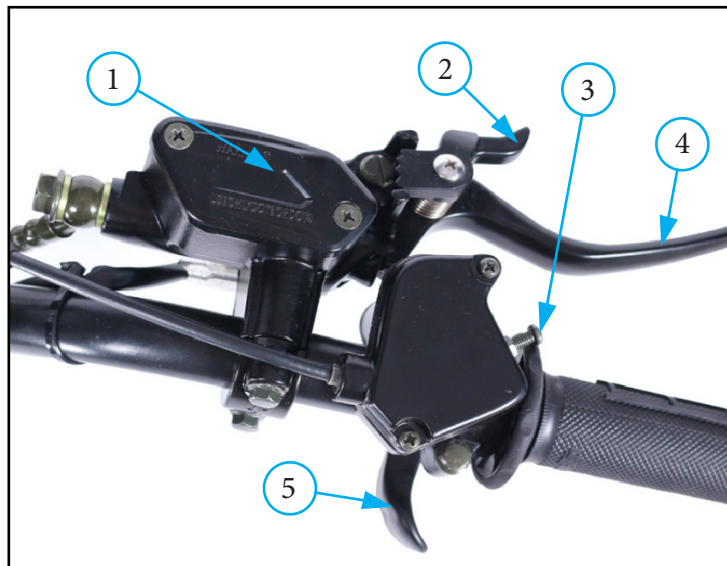
Фото 2.5. Переключатели правого рулевого блока: 1 - бачок переднего тормоза; 2 - фиксатор парковочного тормоза; 3 - регулятор ограничения акселератора; 4 - рычаг переднего тормоза; 5 - рычаг акселератора.
