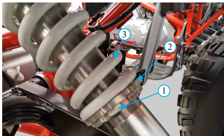
Фото 5.19. Преднатяг пружины заднего амортизатора: 1 – гайка контррочная; 2 – гайка регулировочная; 3 – пружина.
