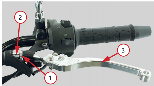
Фото 2.11. Регулировка сцепления: 1 – стопорная гайка; 2 – регулировочный винт; 3 – рычаг сцепления
