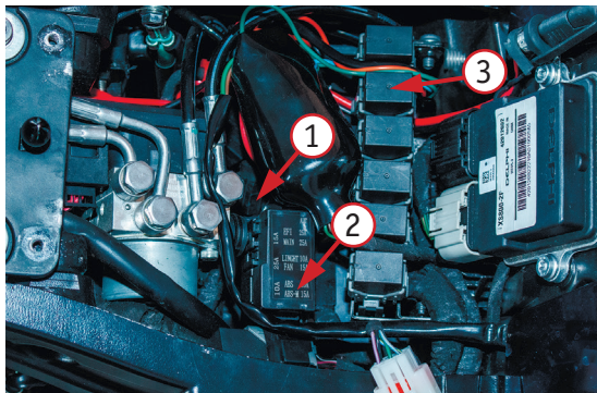
Фото 4. Аккумуляторный отсек: 1 – аккумуляторная батарея (АКБ); 2 – блок предохранителей; 3 – блок реле
