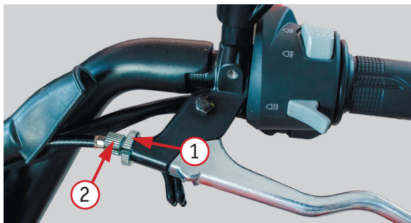
Фото 2.12. Регулировка сцепления: 1 – стопорная гайка; 2 – регулировочный винт
