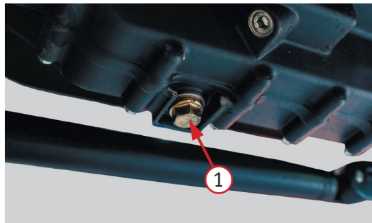
Фото 5.5. Болт слива масла – 1
