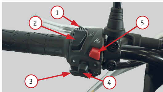
Фото 2.4. Левый комбинированный переключатель: 1 – кнопка включения дальнего света при обгоне; 2 – кнопка переключения режима света фары (дальний свет/ближний свет); 3 – кнопка звукового сигнала; 4 – кнопка указателей поворота; 5 – кнопка включения аварийной сигнализации
