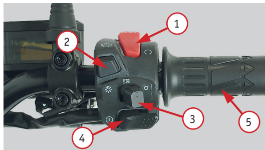
Фото 2.5. Правый комбинированный переключатель: 1 – кнопка включения/отключения питания; 2 – кнопка ABS, кнопка включения/выключения света; 3 – включить освещение; 4 – электростартер; 5 – ручка газа (акселератора)
