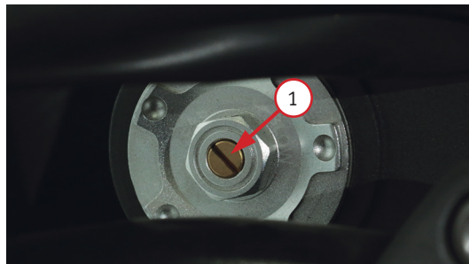
Фото 2.14. Регулировка демпфирования переднего и заднего амортизатора: регулировочный винт - 1
