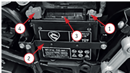
Фото 4. Аккумуляторный отсек и блок предохранителей: 1 – клемма «минус»; 2 – крепежная пластина аккумуляторной батареи (АКБ); 3 – аккумуляторная батарея; 4 – клемма «плюс»
