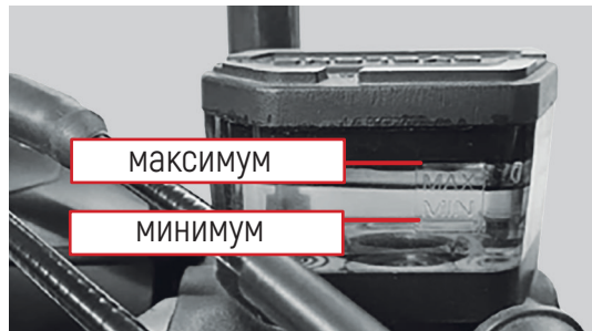
Фото 5.8. Бачок тормозной жидкости передних тормозов
